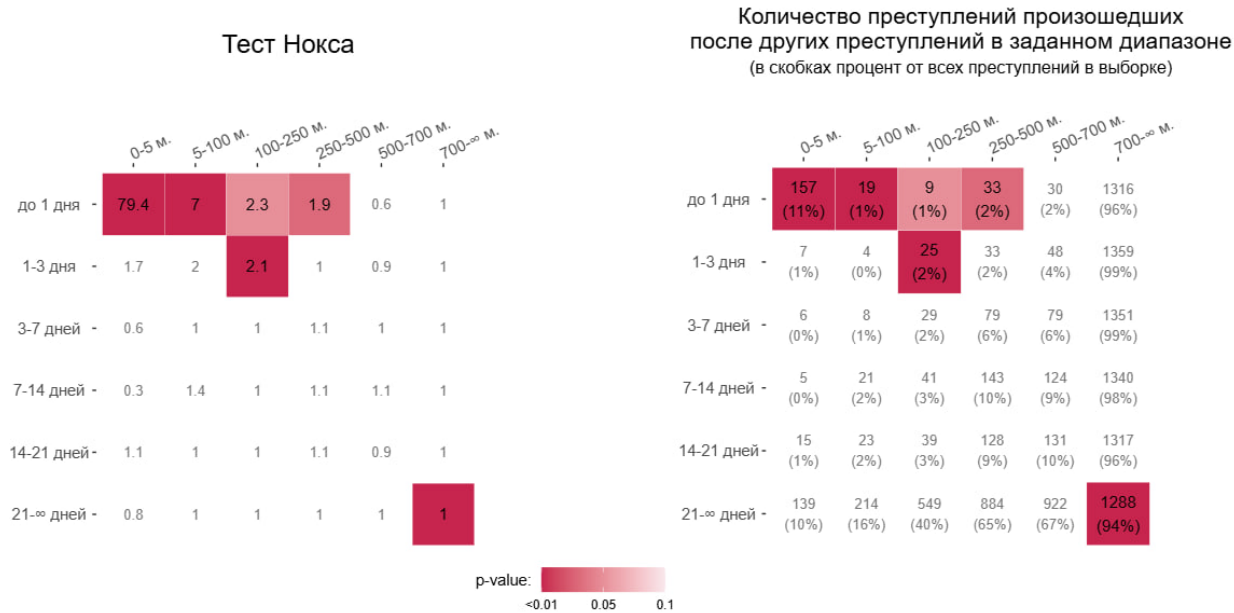
Рисунок 7. Тест Нокса для всех насильственных преступлений* г. Алматы**
