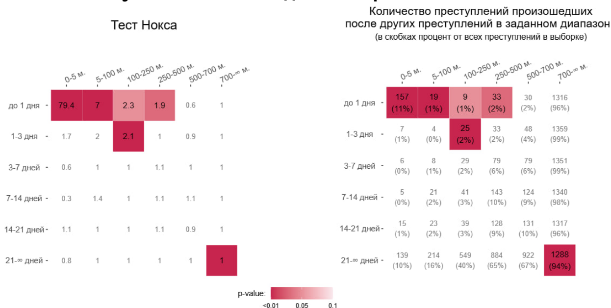
Рисунок 5. Тест Нокса для всех краж* г. Алматы**
