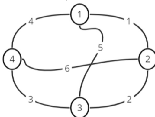
Рисунок 1. Иллюстрация максимального числа пар между событиями
